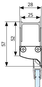
Wandprofil Magnetanschlag 6 mm Glas flächenbündig Aluminium
