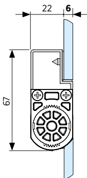
Drehprofil Glas-Glas 6 mm Glas flächenbündig Hebe-/Senkmechanismus Aluminium
