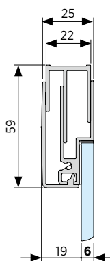
Wandanschlussprofil flächenbündig 6 mm Glas Aluminium
