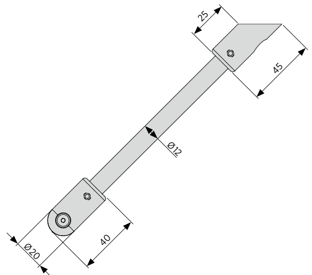
45°-Stabilisator, rund (rechts) 6 mm Glas Aluminium und Messing, verchromt
