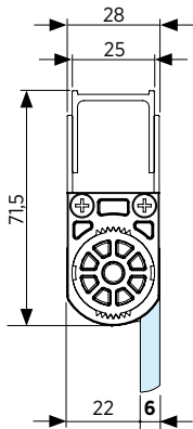
Drehprofil Wand-Glas 6 mm Glas flächenbündig (links) Hebe-/Senkmechanismus Aluminium
