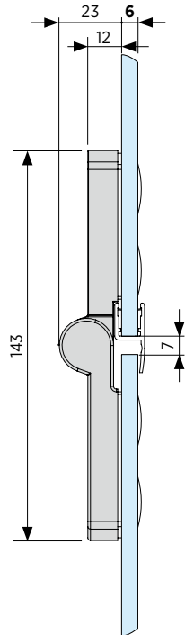
Scharnier Glas-Glas 6 mm Glas Hebe-/Senkmechanismus Messing, verchromt
