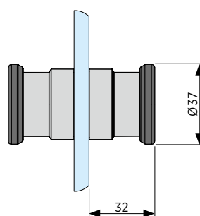
⑧ Rundgriff verschraubt 6 mm Glas Zinkdruckguss, verchromt
