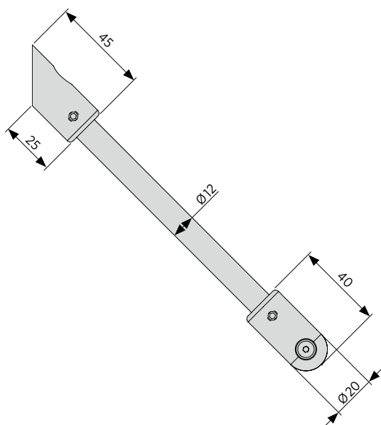
② 45°-Stabilisator, rund (links) 6 mm Glas Aluminium und Messing, verchromt
