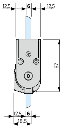
⑦ Drehprofil Glas-Glas (links) 6 mm Glas Hebe-/Senkmechanismus Aluminium
