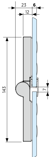
⑤ Scharnier Glas-Glas 6 mm Glas Hebe-/Senkmechanismus Zinkdruckguss, verchromt
