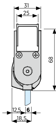
⑥ Drehprofil Wand-Glas (links) 6 mm Glas Hebe-/Senkmechanismus Aluminium
